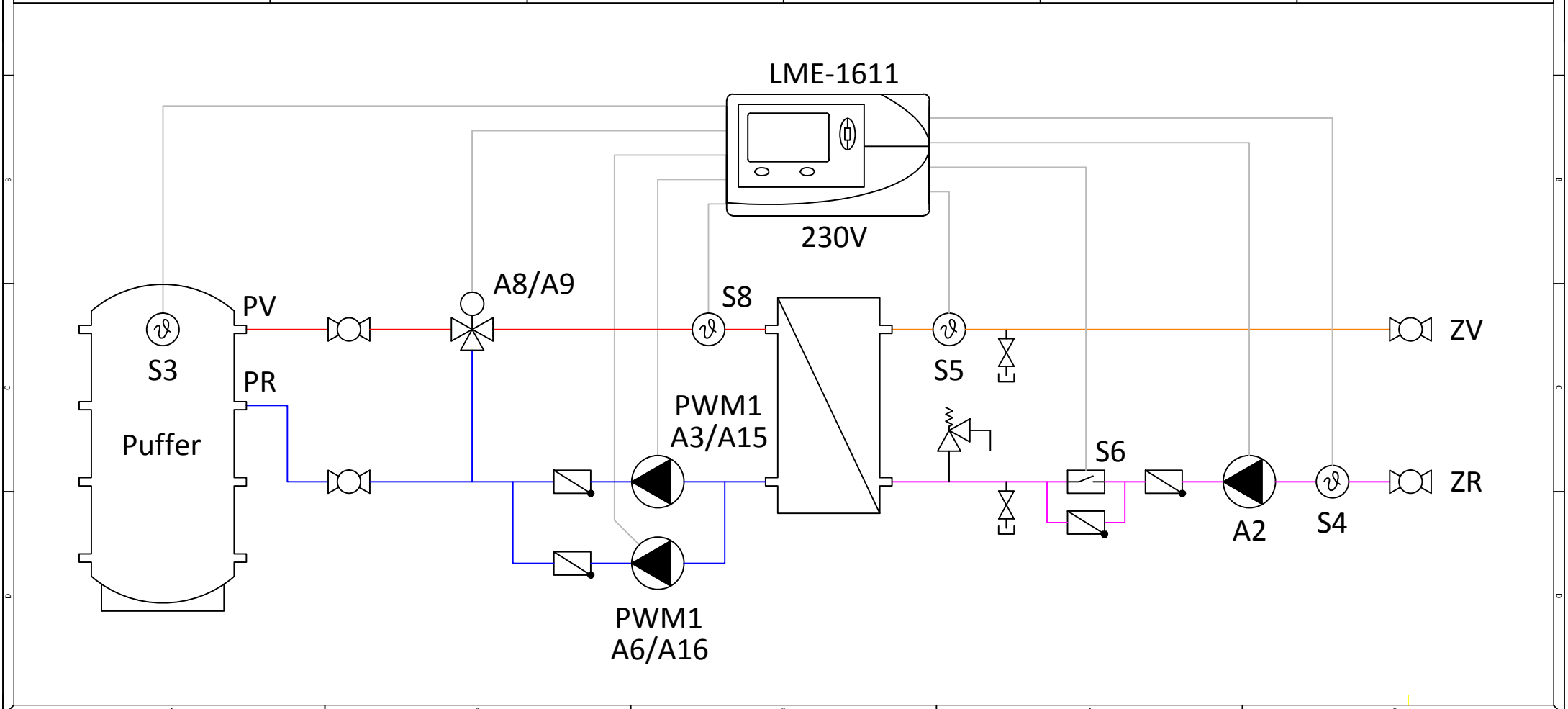
LME | Hydraulikschemata | Zirkulationsmodul | 30 kW bis 50 kW
