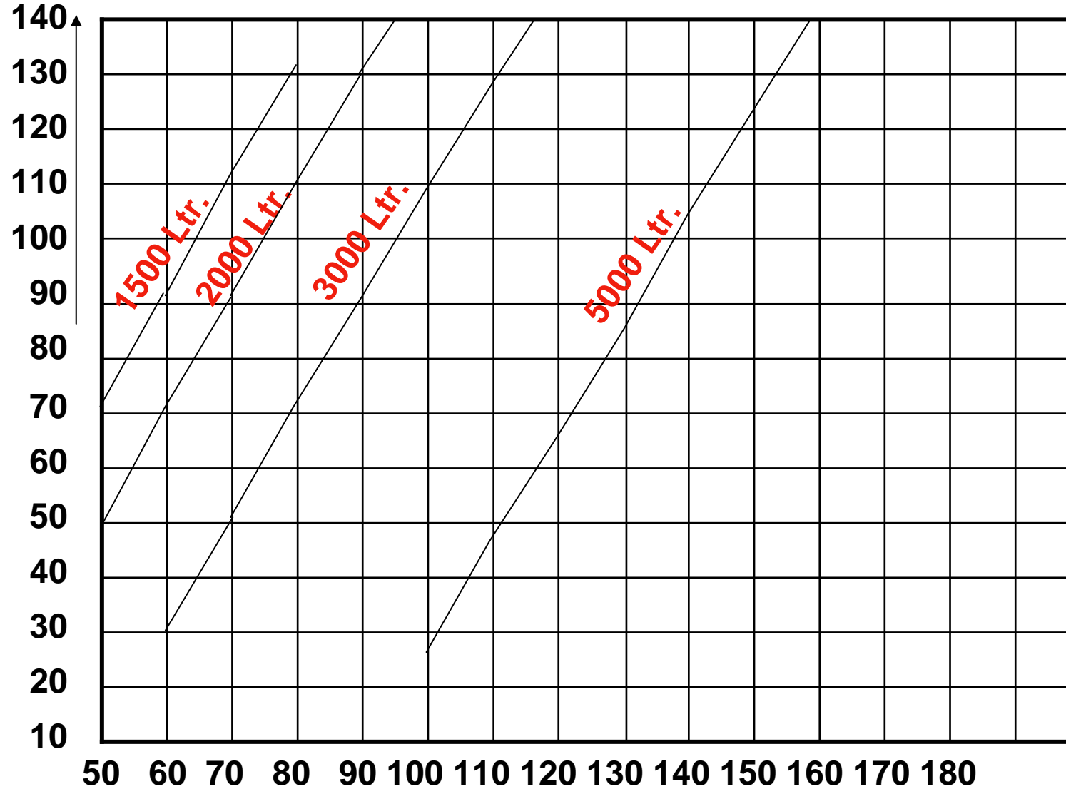
Dimensionierung Zusatzleistung Warmwasser 15l/min
