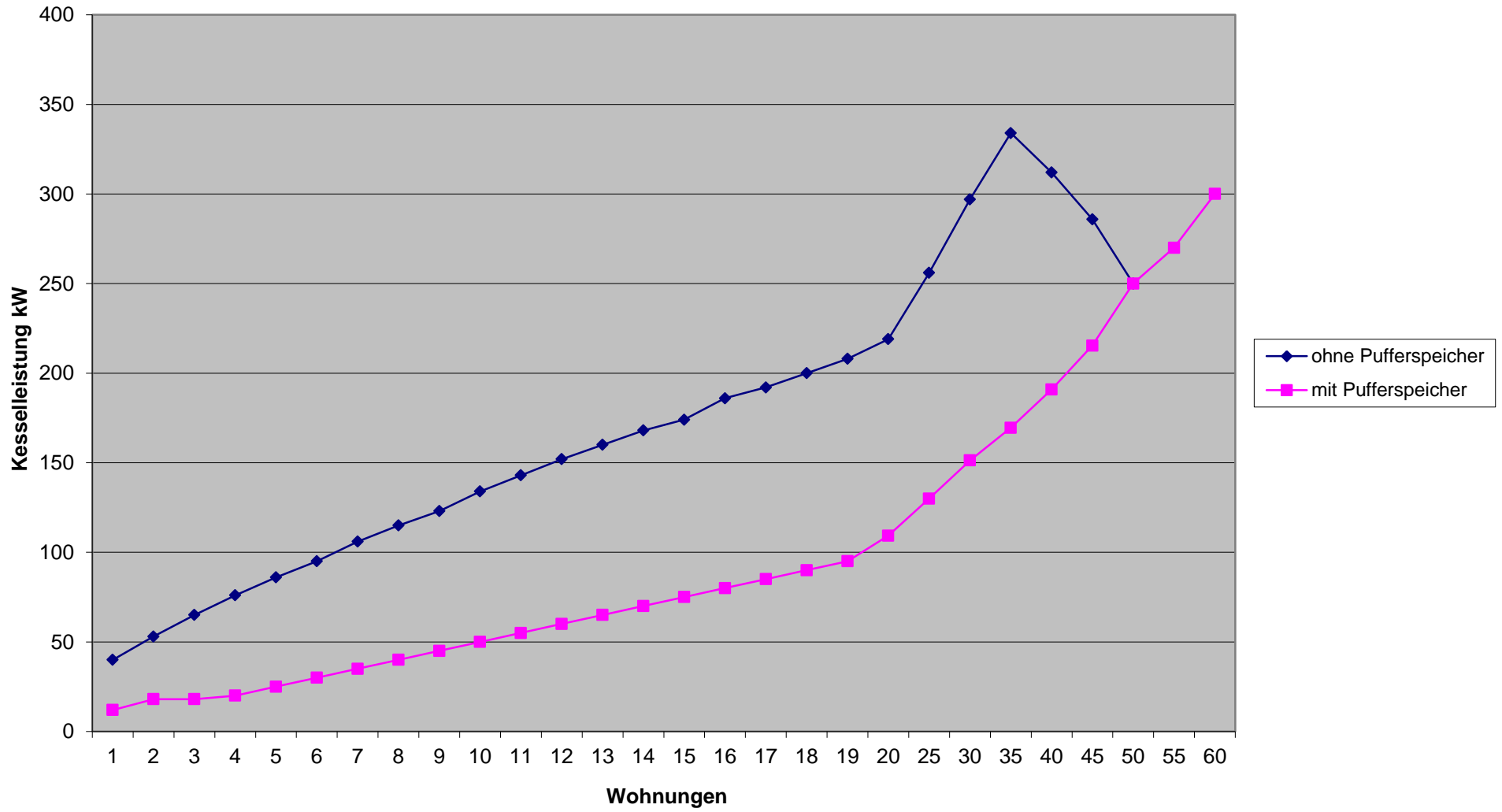
Kesselleistung bei 5kW Heizleistung, 35kW Warmwasser
