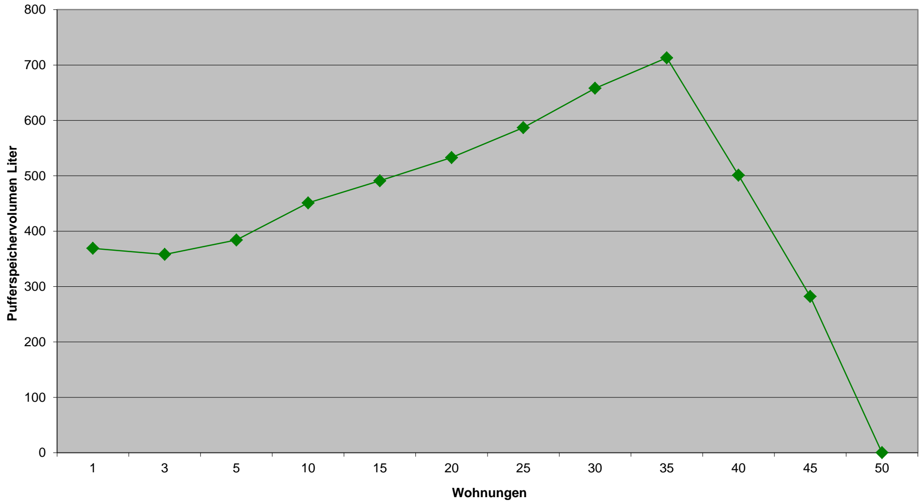
Pufferspeichervolumen bei 5kW Heizleistung, 35kW Warmwasser
