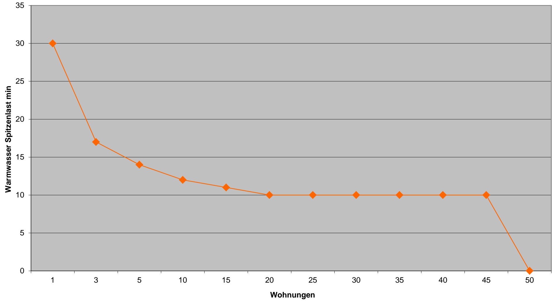
Warmwasserspitzenlast bei 5kW Heizleistung, 35kW Warmwasser
