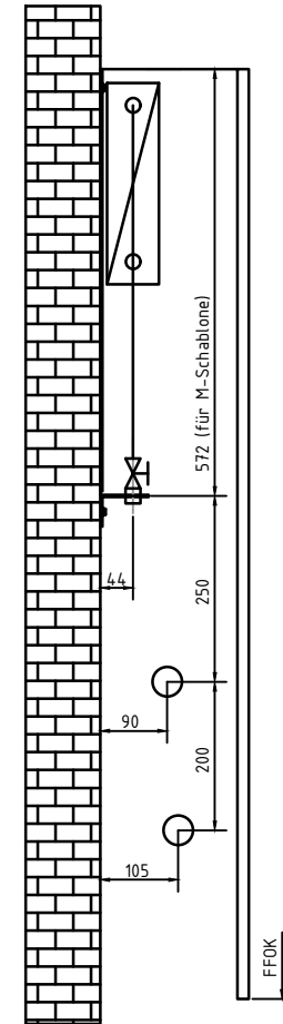
LME | Maßskizzen | LME-APOU 1250x800x200 mm | Wohnungsstation für FB-Heizung mit Festwertregelung, 2-10 FB-Kreise, 36/45/55 kW mit Abdeckhaube unten offen
