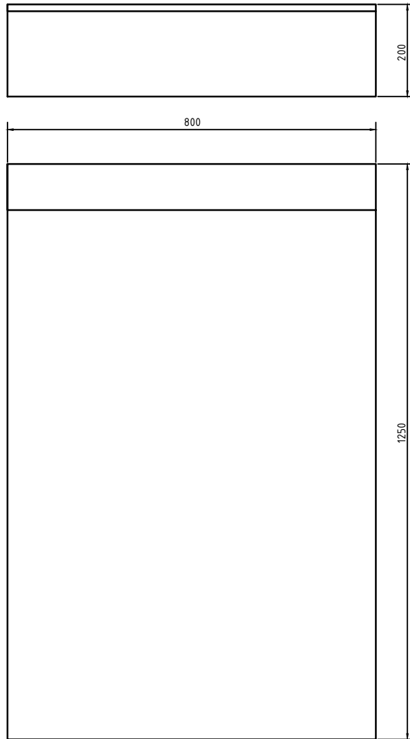
LME | Maßskizzen | LME-APOU 1250x800x200 mm | Wohnungsstation für FB-Heizung mit Festwertregelung, 2-10 FB-Kreise, 36/45/55 kW mit Abdeckhaube unten offen
