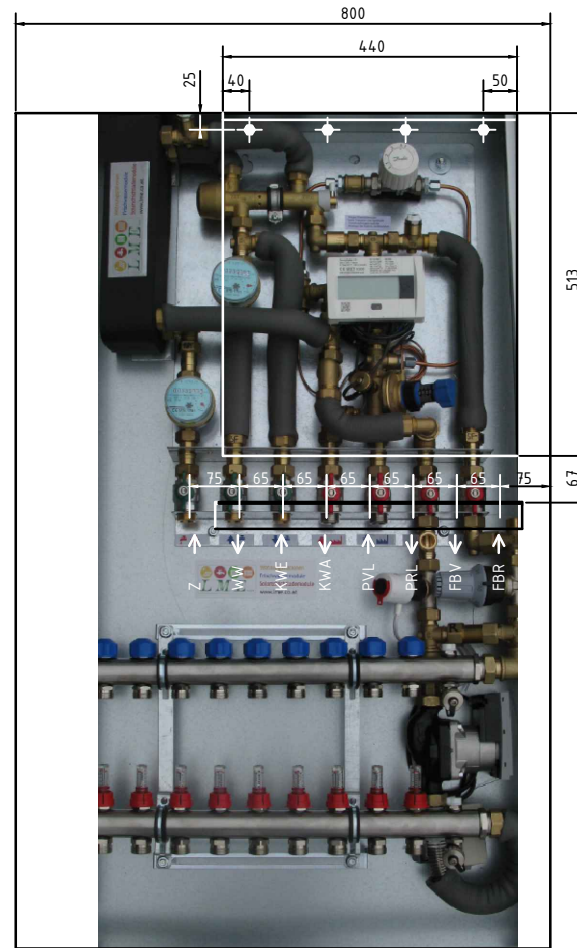
LME | Maßskizzen | LME-APOU 1250x800x200 mm | Wohnungsstation für FB-Heizung mit Festwertregelung, 2-10 FB-Kreise, 36/45/55 kW mit Abdeckhaube unten offen
