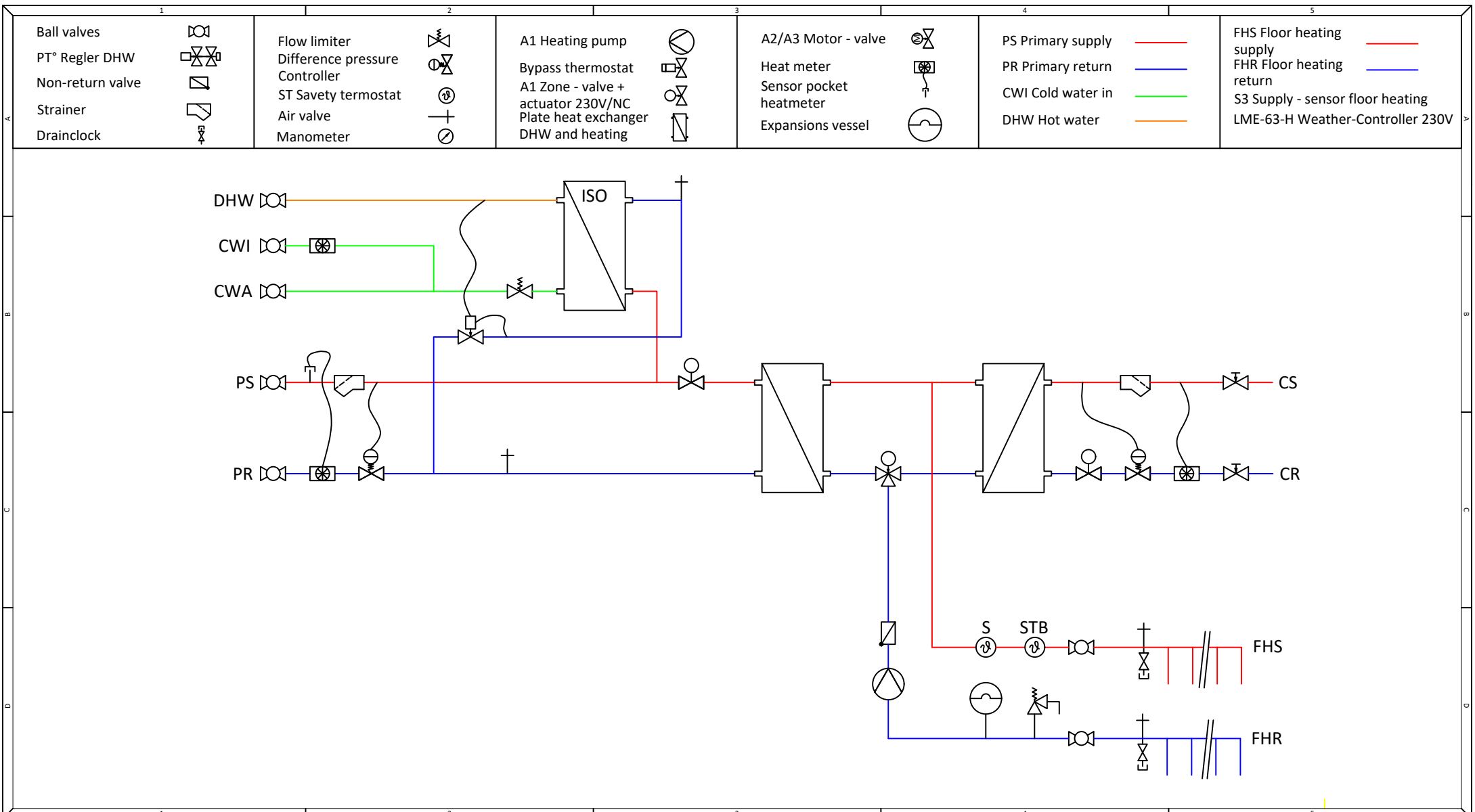
LME | Hydraulic - diagram | Wohnungsstation mit indirekter Heizung und Kühlung und Warmwasser
