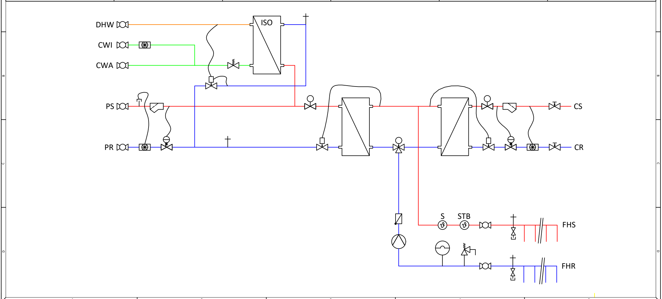
LME | Hydraulic - diagram | Wohnungsstation mit indirekter Heizung und Kühlung mit Festwertregelung und Warmwasser
