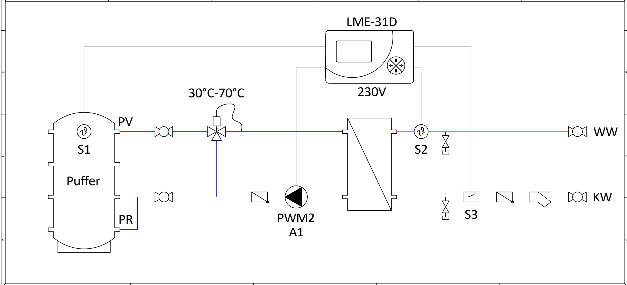
LME | Hydraulikschemata | Frischwassermodul ohne Zirkulation und ohne Rücklaufumschaltung | 26 Liter bis 35 Liter
