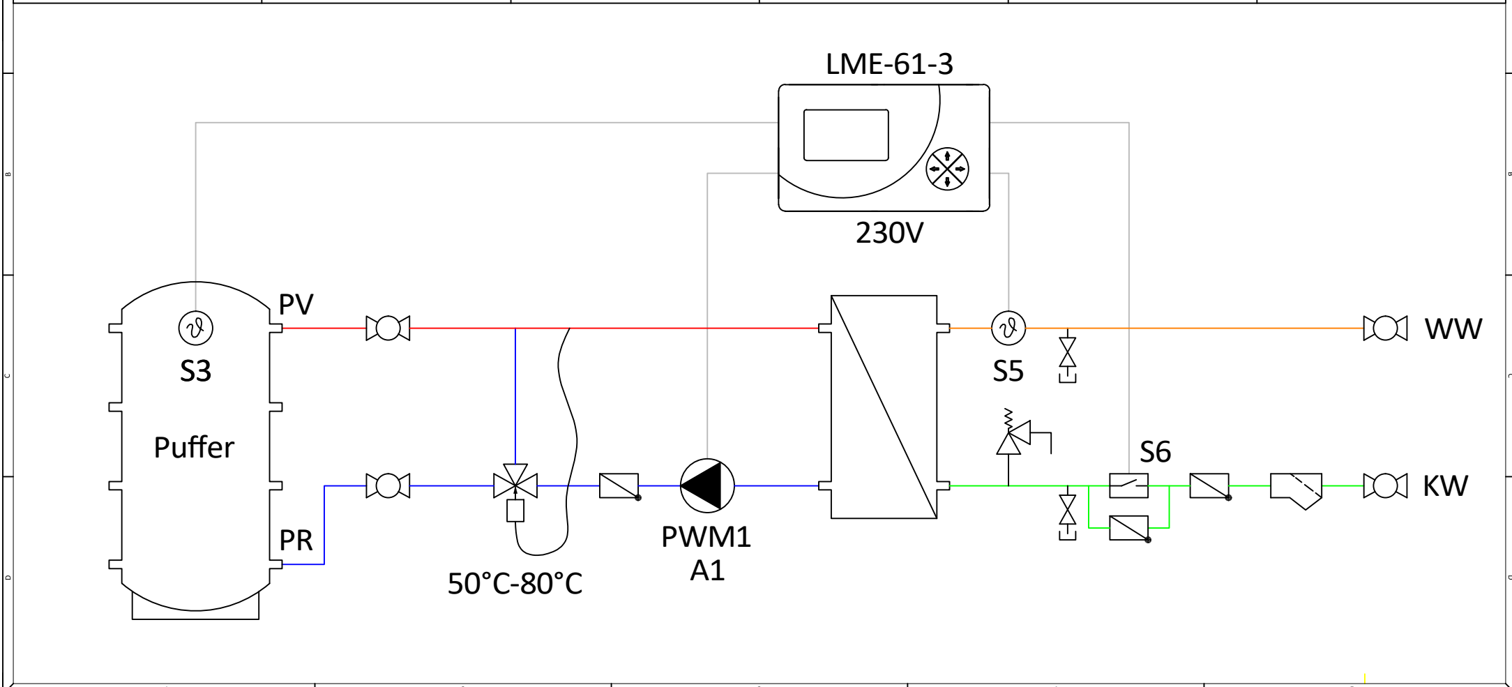
LME | Hydraulikschemata | Frischwassermodul ohne Zirkulation und ohne Rücklaufumschaltung | 50 Liter bis 115 Liter
