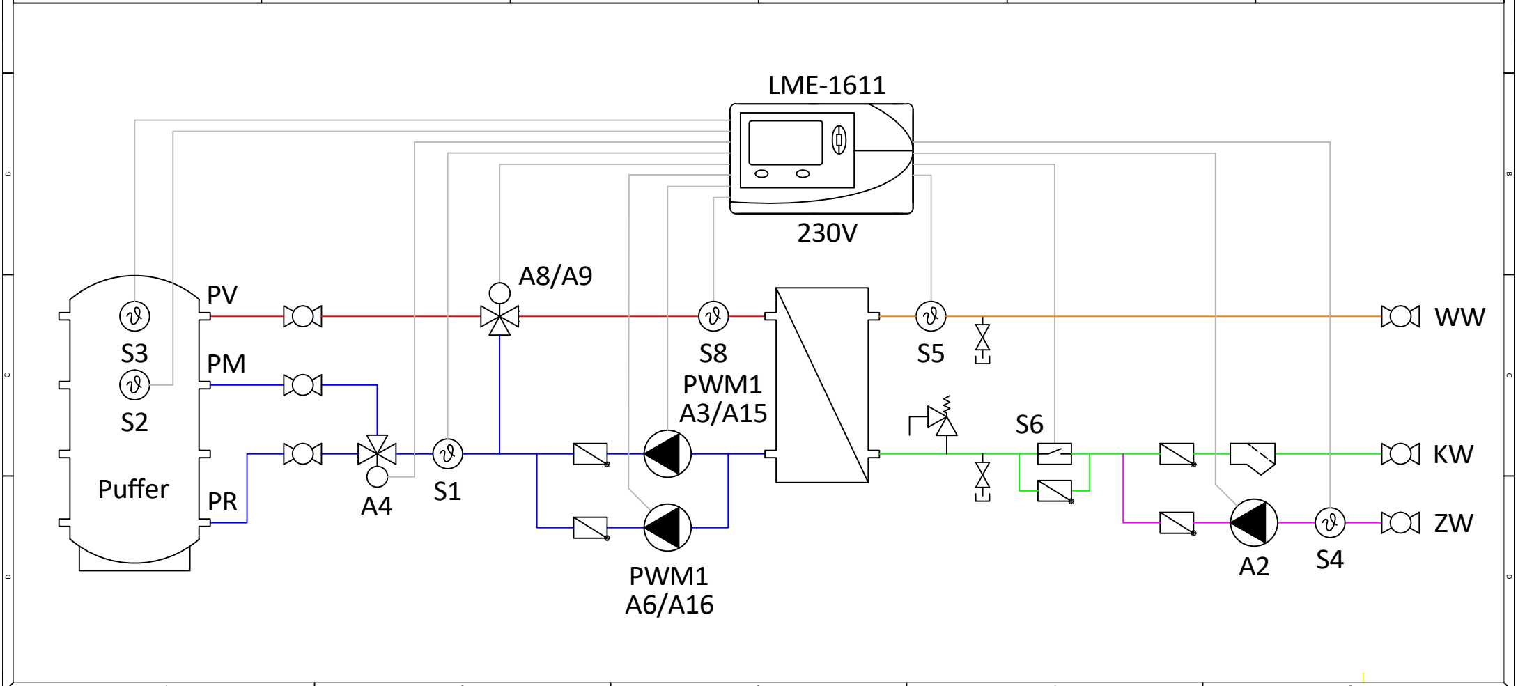
LME | Hydraulikschema | Frischwassermodule mit Zirkulation und mit Rücklaufumschaltung | 150 Liter bis 250 Liter
