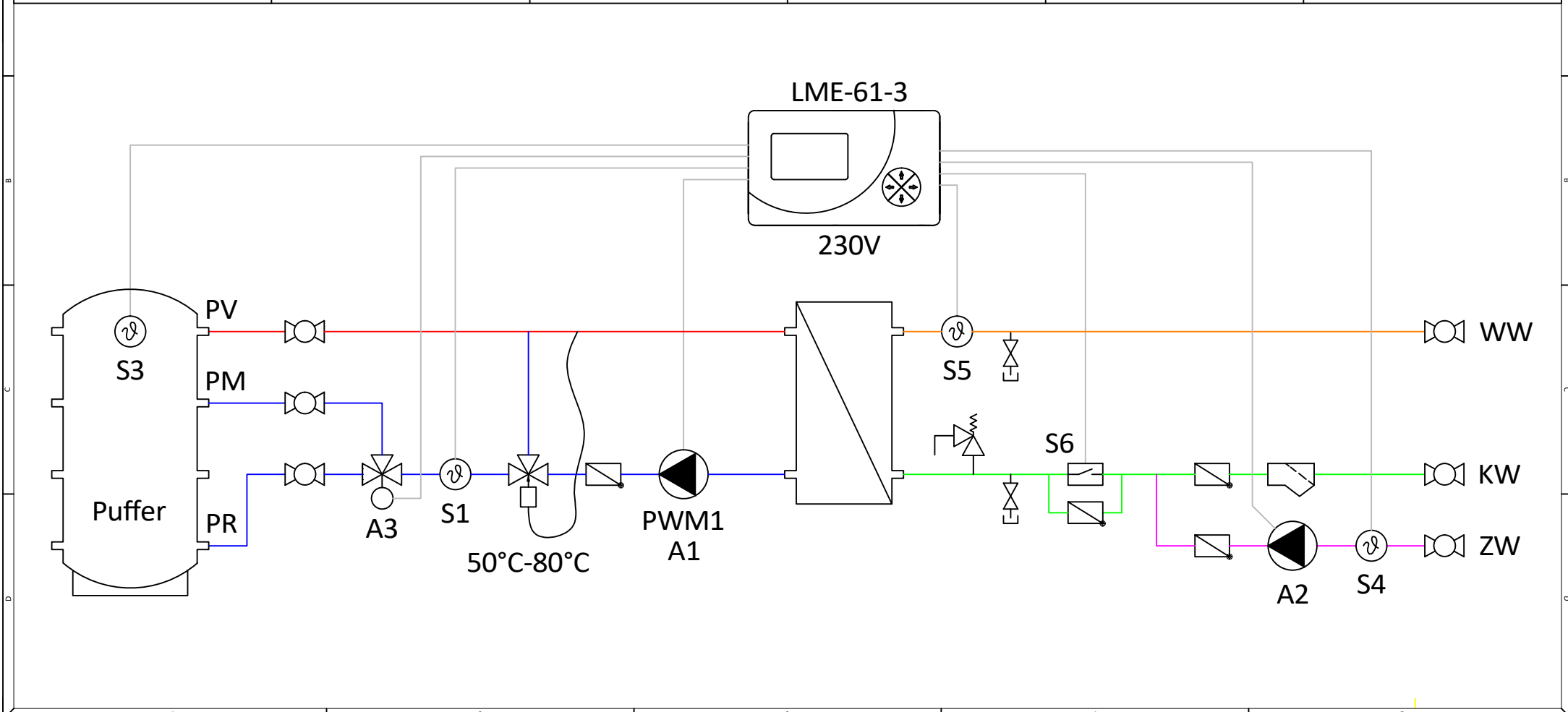
LME | Hydraulikschemata | Frischwassermodul mit Zirkulation und mit Rücklaufumschaltung | 50 Liter bis 115 Liter
