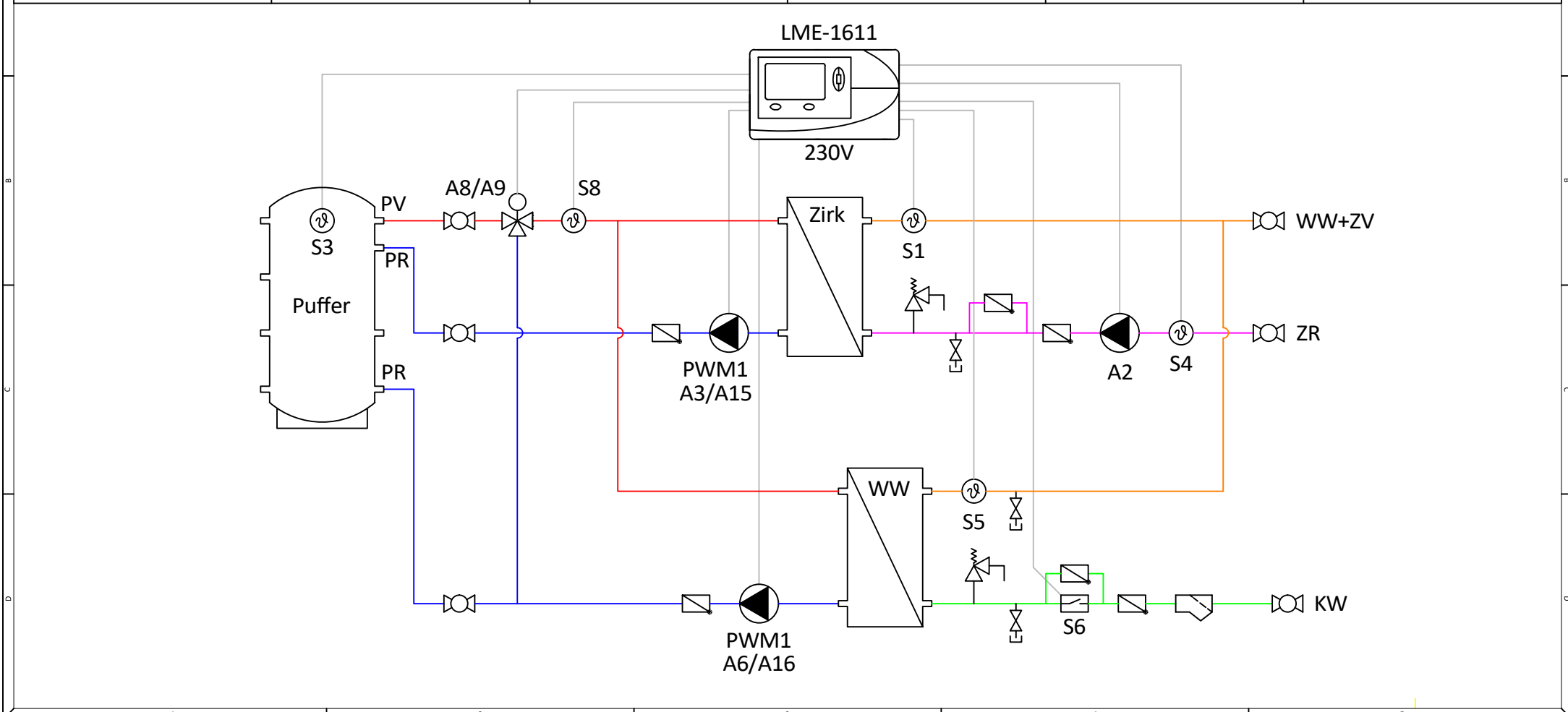
LME | Hydraulikschemata | Frischwassermodul 50-115 Liter mit Zirkulationsmodul 5-20kW
