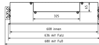
A-A (1:5)
