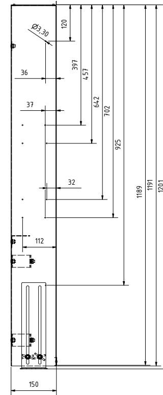
A-A (1:5)
