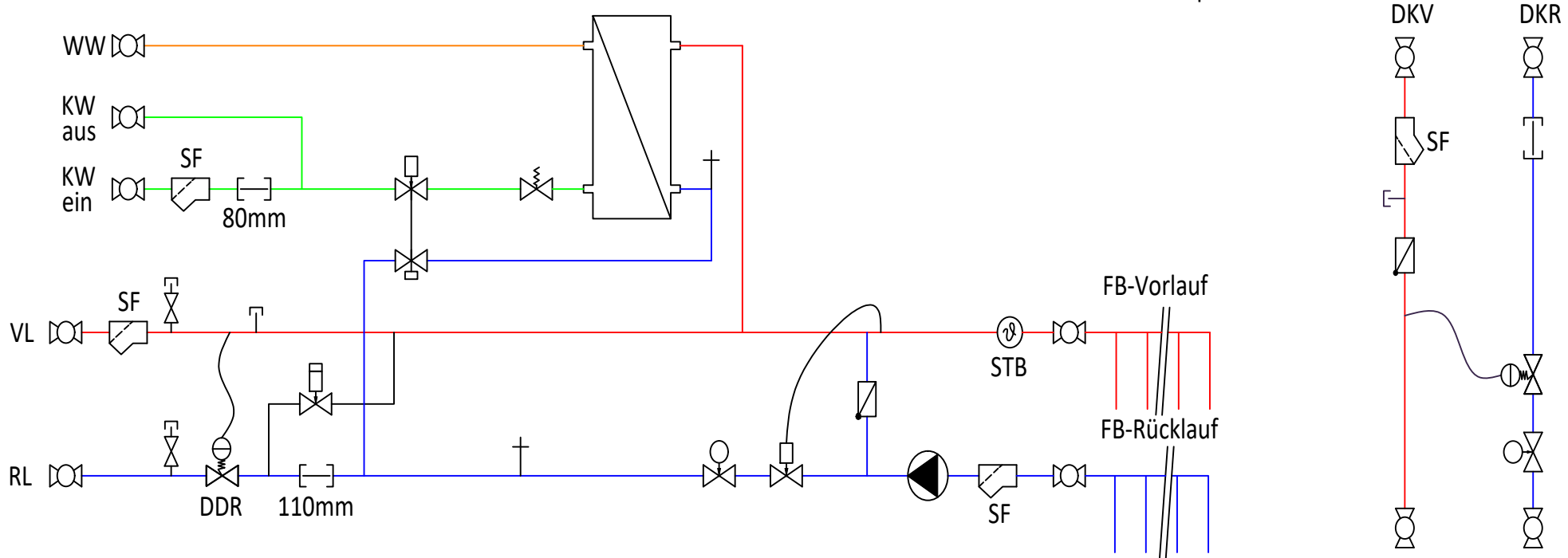
LME | Hydraulikschemata | Wohnungsstation für Warmwasser, Fußbodenheizung mit Festwertregelung und direkte Deckenkühlung
